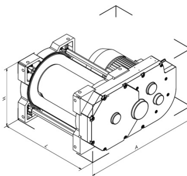
TRBoxter 250 à 990 kg – commande directe
