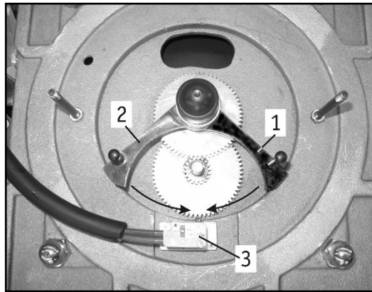
B. Fin de course type à came IP65
